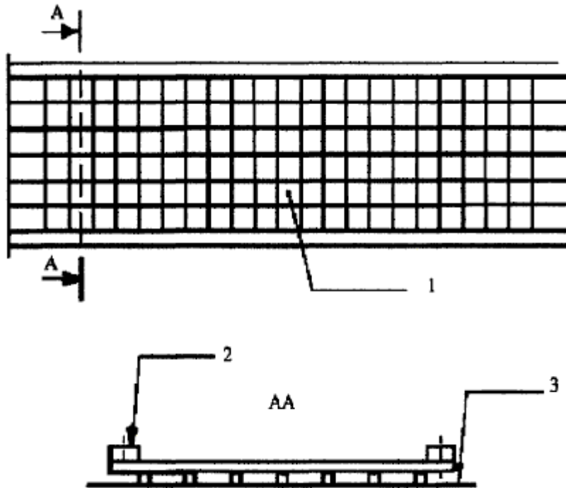
Фигура 8 Елемент от конструкцията и монтаж на пистата за движение
