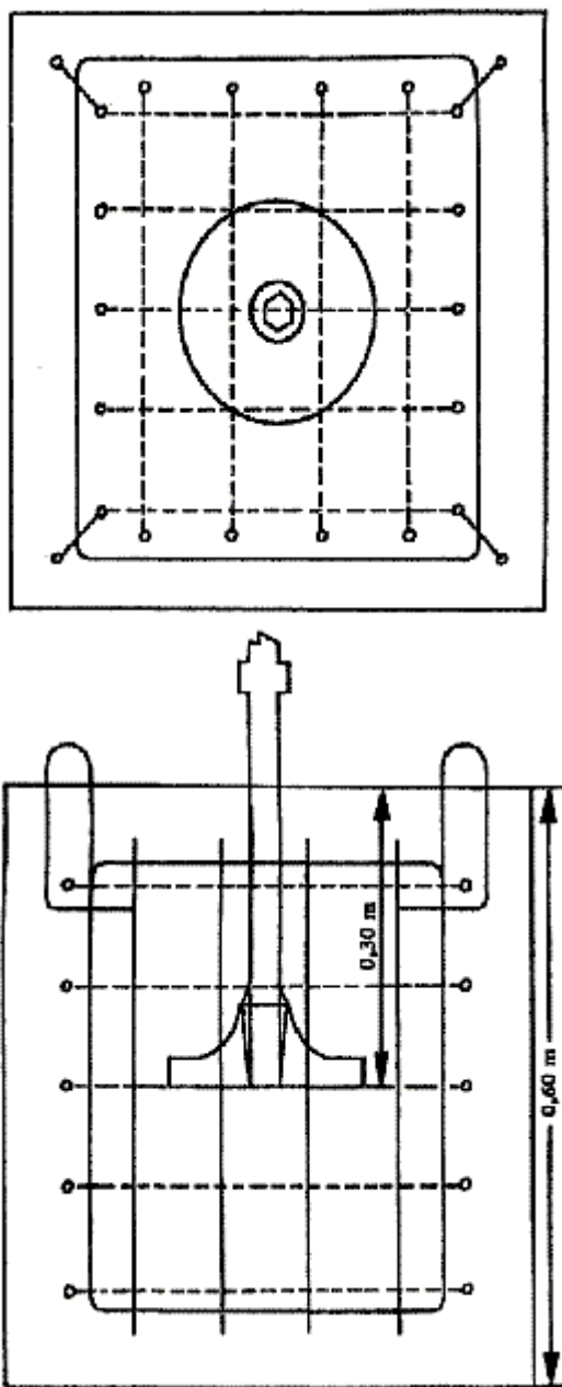
Фигура 3 Блок за изпитване
