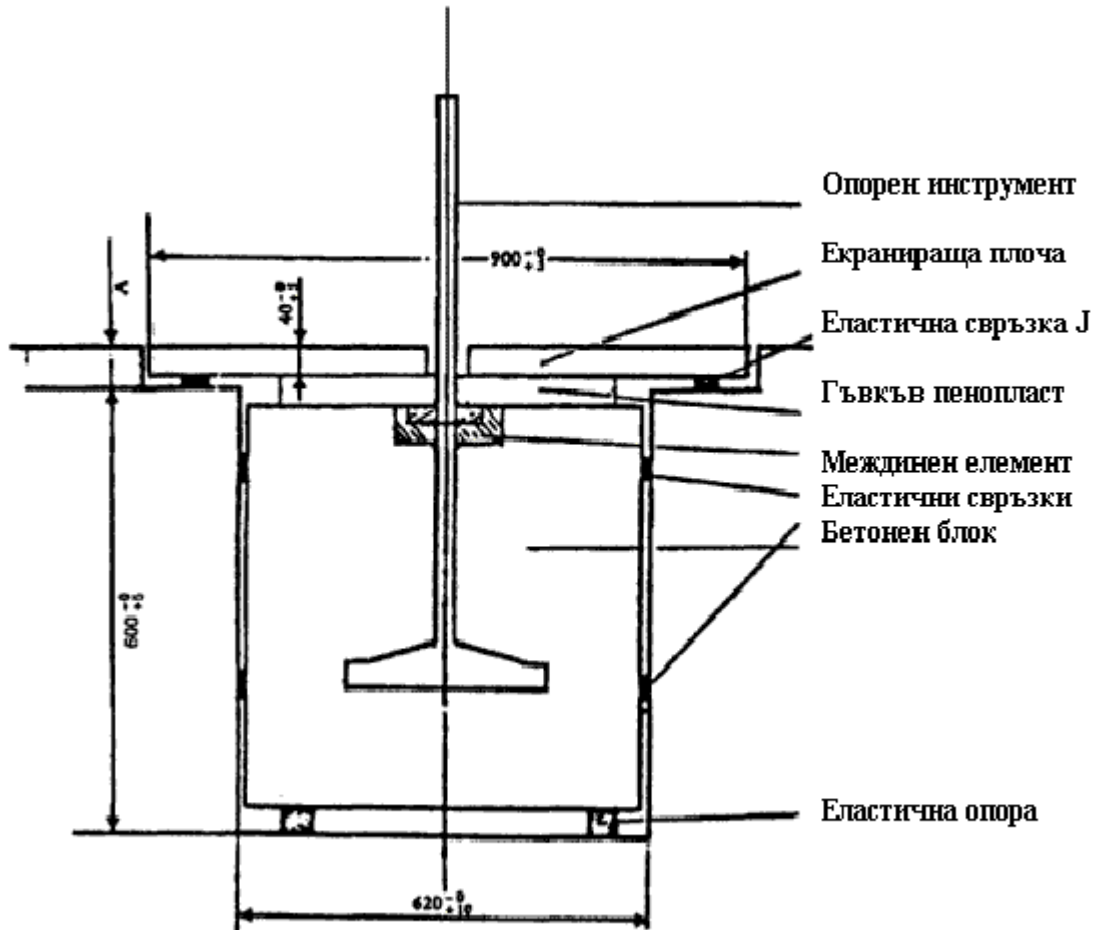
Фигура 4 Устройство за изпитване
